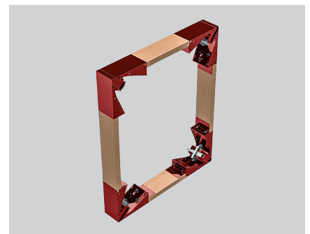
Kevyet ja korkealaatuisella pulverimaalauksella käsitellyt alumiiniosat varmistavat suorakulmaiset ja kohtisuorat aukkovaraukset.
