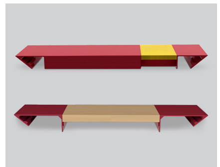
Multi- ja VARIO-elementtien avulla voidaan tehdä monenlaisia oven ja ikkunan leveydenhienosäätöjä.
