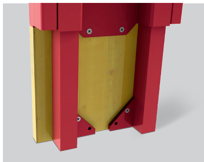
Teleskooppisäätömahdollisuuden ansiosta ovikorkeutta voidaan säätää 200–250 cm:n välillä.
